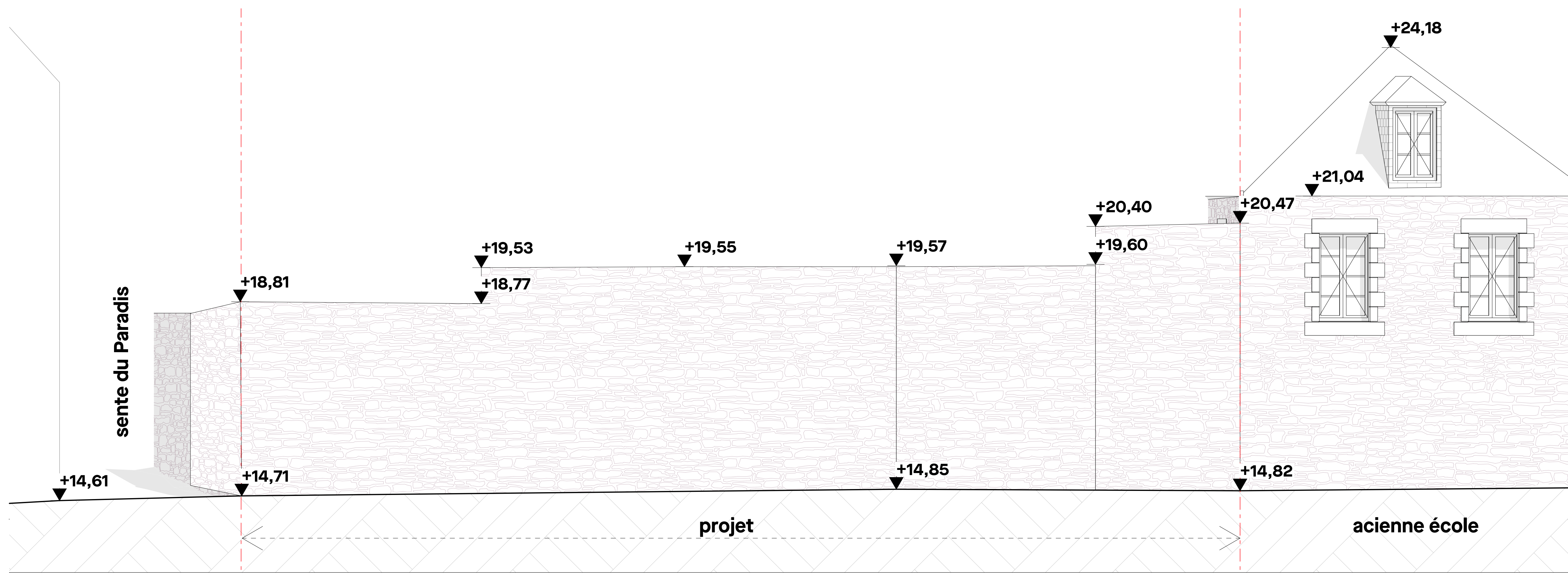
F09 - Elévation mur de clôture sur rue des Anciennes Ecoles
