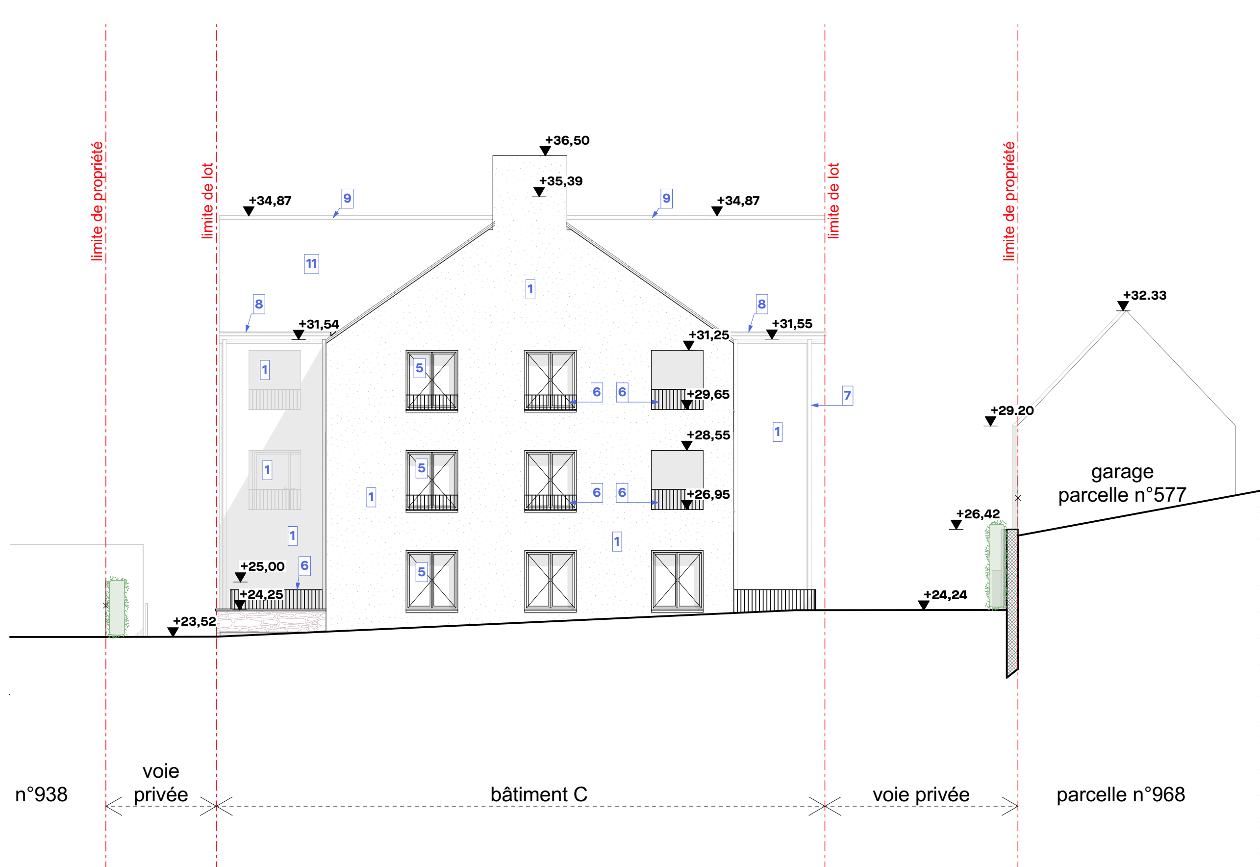
F04 - Bâtiment C - Façade Ouest
