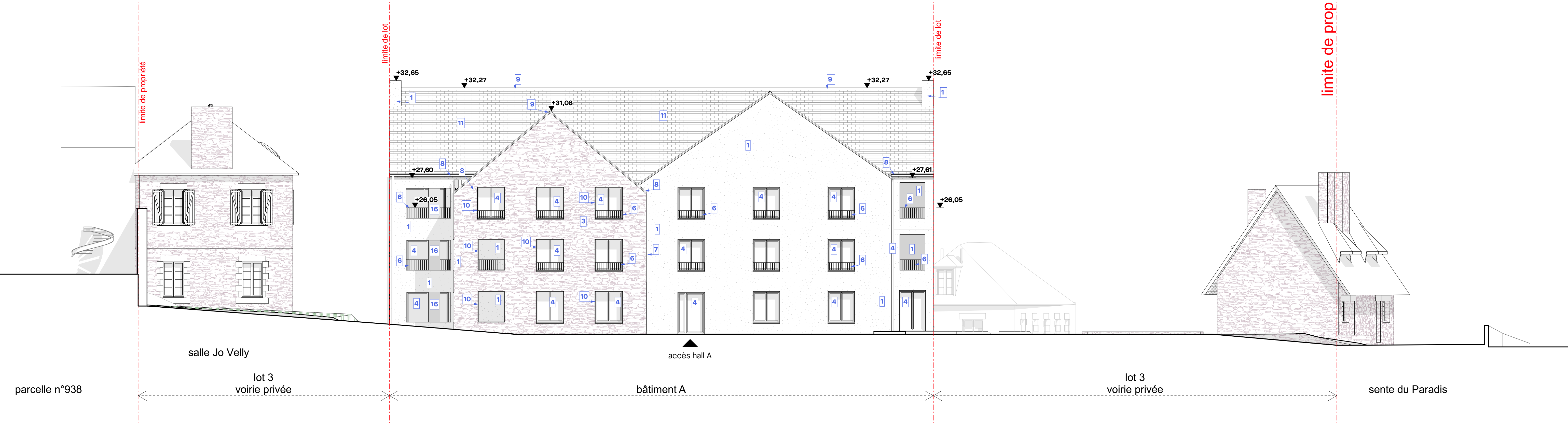
F05 - Bâtiment A - Façade Sud
